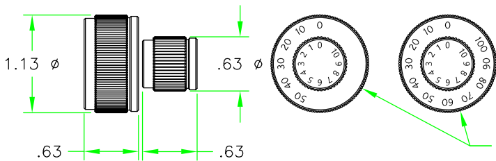
DETAIL A: KNOB DETAILS
